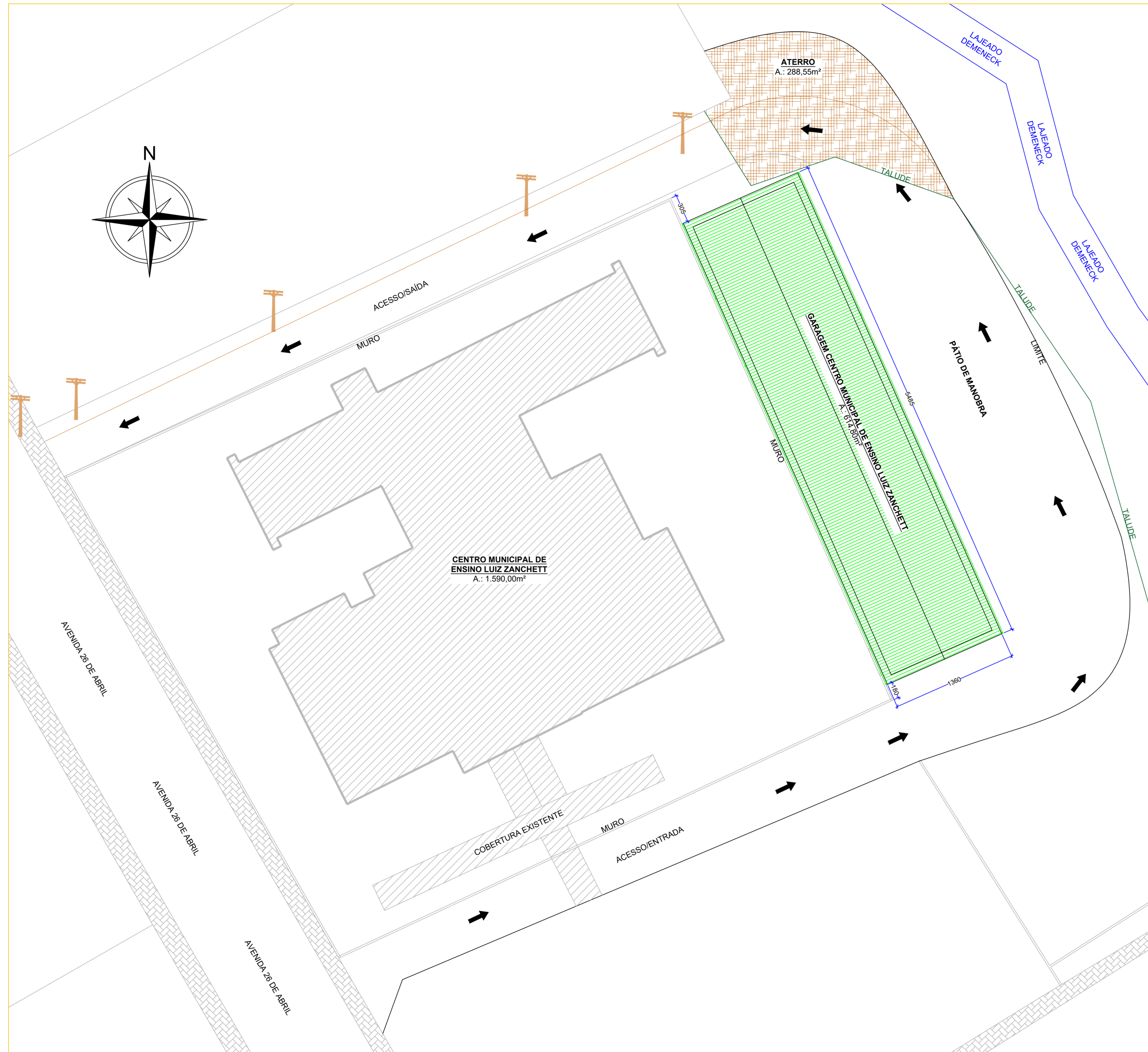
PLANTA DE LOCAÇÃO E SITUAÇÃO GARAGEM CENTRO MUNICIPAL DE ENSINO LUIZ ZANCHETT A.: 614,80m 2 Esc.: 1:250
