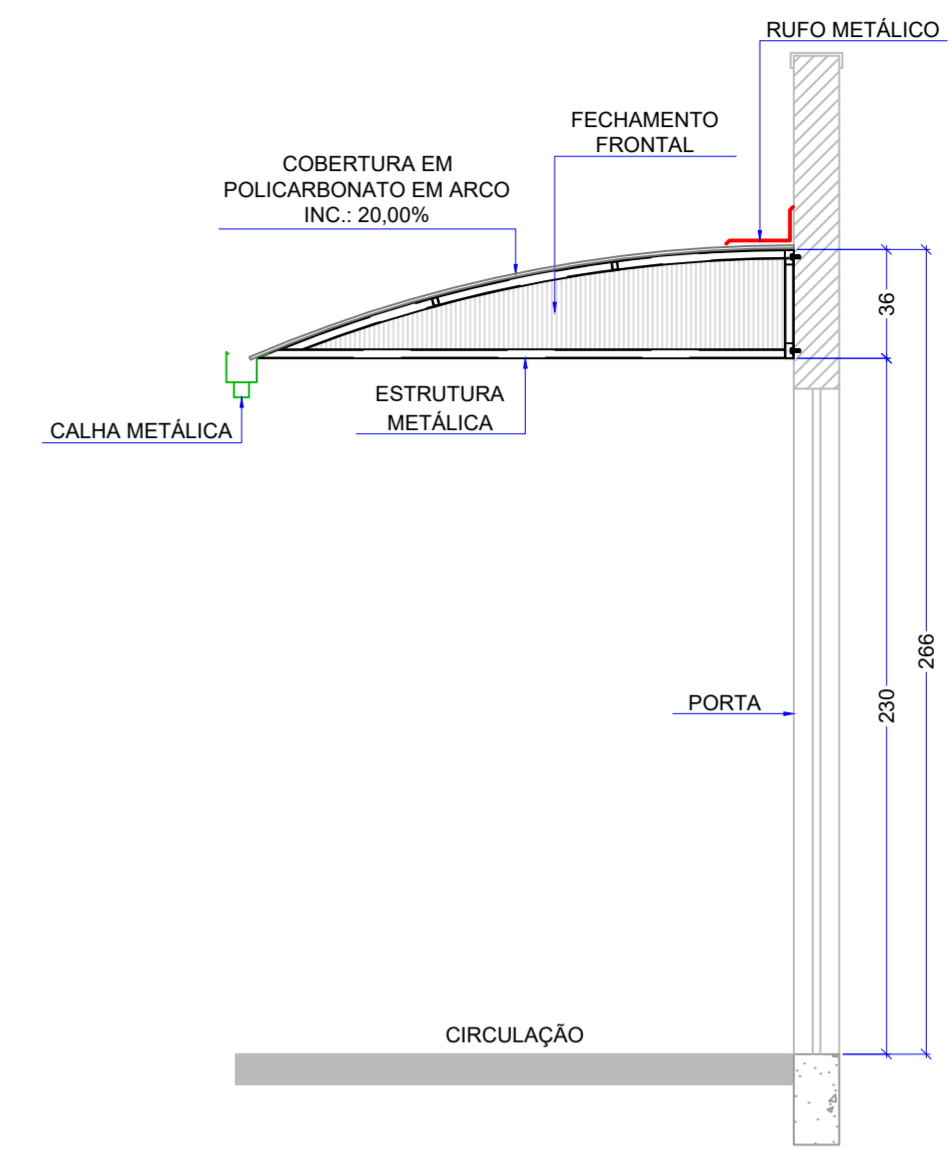
CORTE "D-D" - FACHADA FUNDOS (ACESSO COZINHA) Esc.: 1:25
