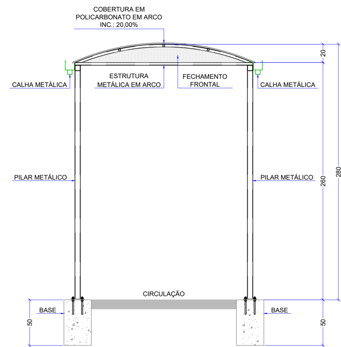
CORTE "C-C" - FACHADA FUNDOS (ACESSO ALUNOS) Esc.: 1:25
