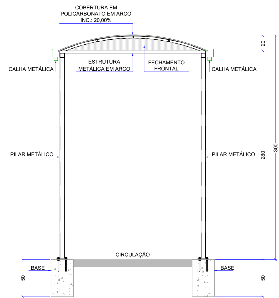
CORTE "A-A" - FACHADA FRONTAL (ACESSO PRINCIPAL) Esc.: 1:25
