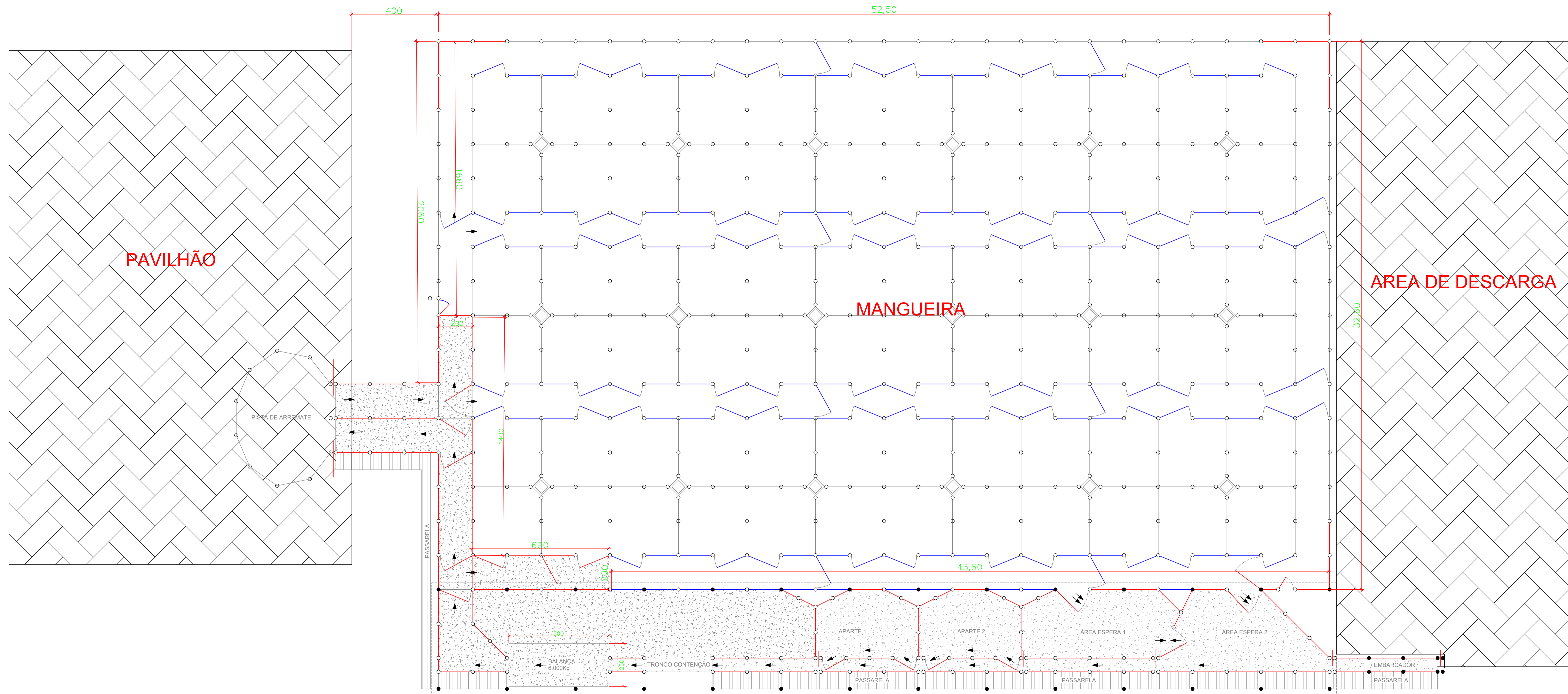
PLANTA BAIXA ESCALA 1:100
