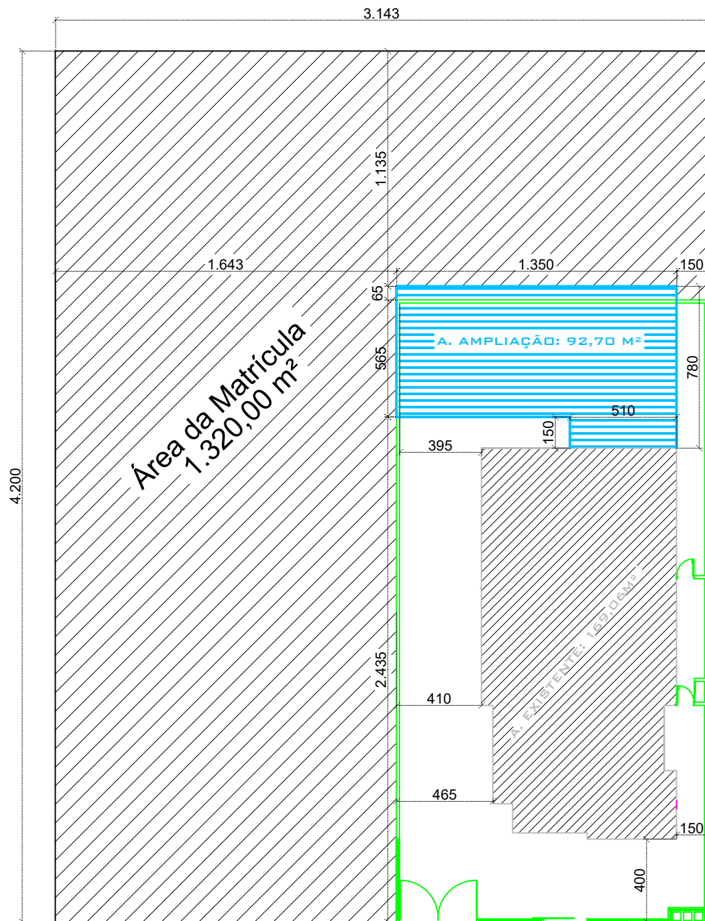
PLANTA DE LOCAÇÃO ESCALA 1:250
