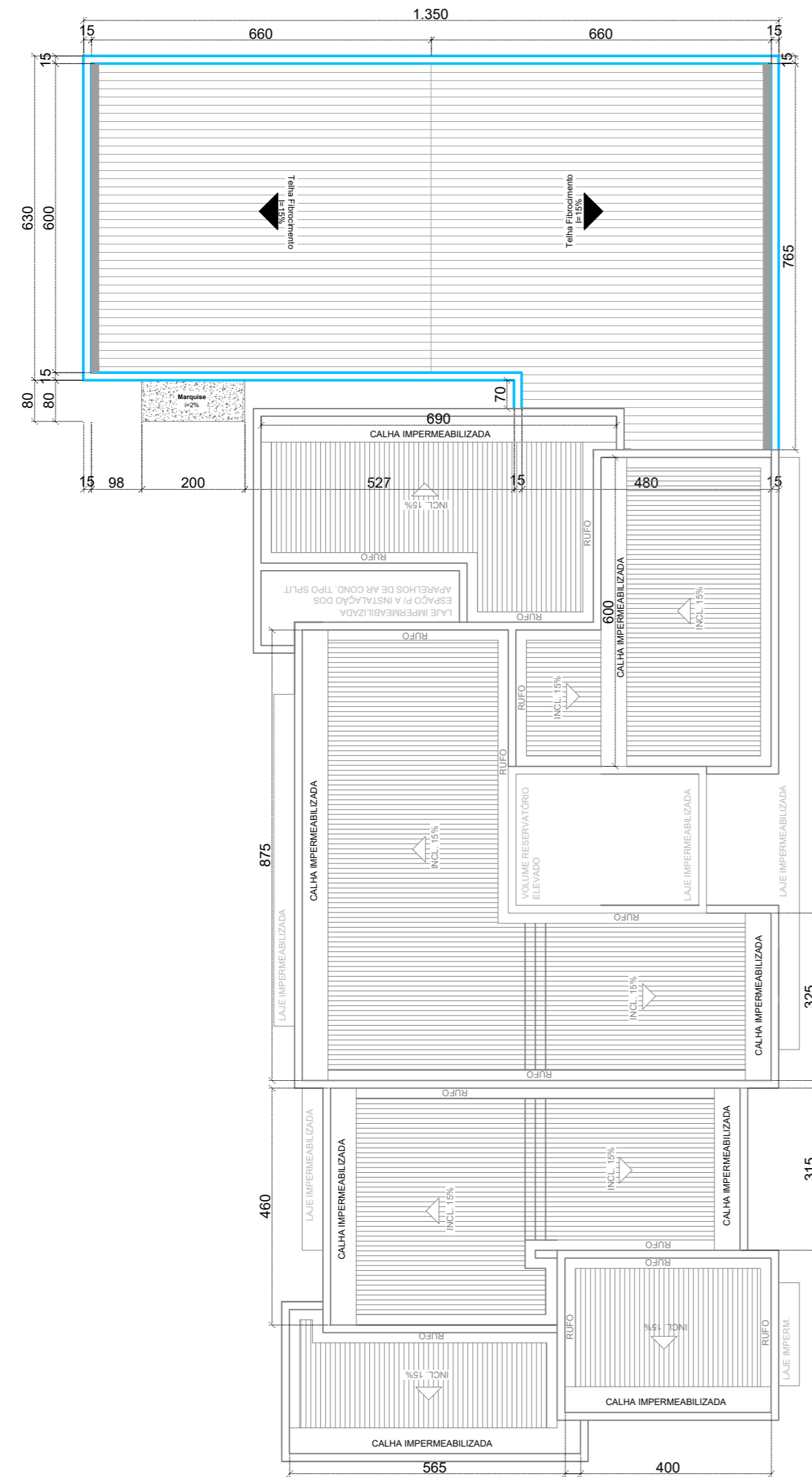
COBERTURA ESCALA 1:100
