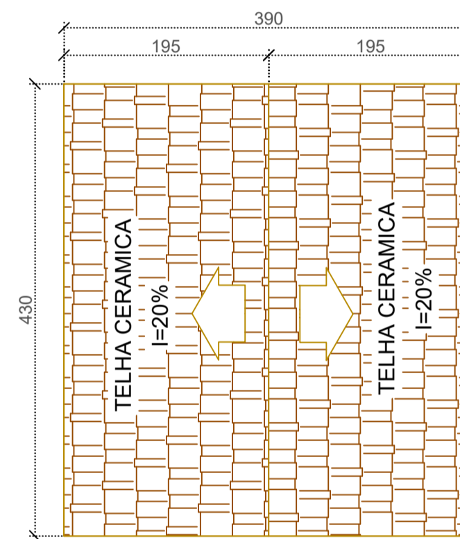
PLANTA DE COBERTURA Esc.: 1:50
