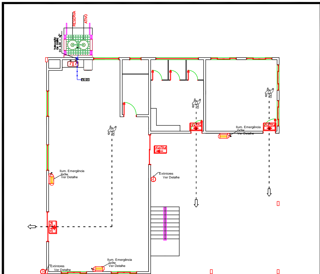
PLANO DE FUGA SEM ESCALA
