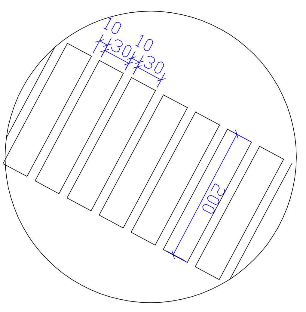
Detalle - Faixa de Pedestres S/ Escala
