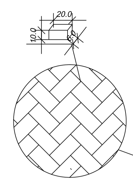
Detalhamento do Paver 10x20x6
