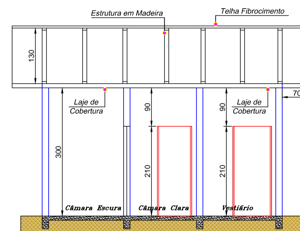
Corte A-A - Ampliação ÁREA= 14,84 M 2 ESCALA ..... 1 : 75
