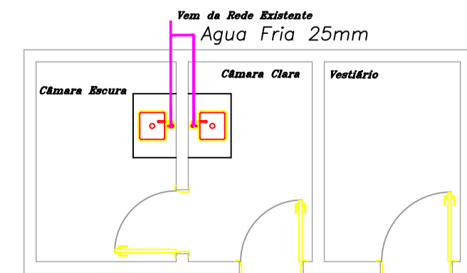
Projeto Hidráulico ÁREA= 14,84 M 2 ESCALA ..... 1 : 75
