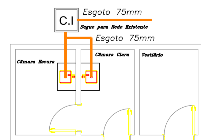
Projeto Sanitário ÁREA= 14,84 M 2 ESCALA ..... 1 : 75
