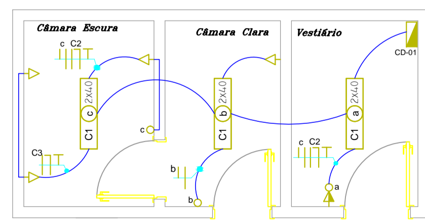
Projeto Elétrico ÁREA= 14,84 M 2 ESCALA ..... 1 : 75
