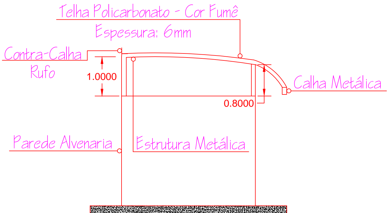
Vista Lateral - Solarium 01 e 02
