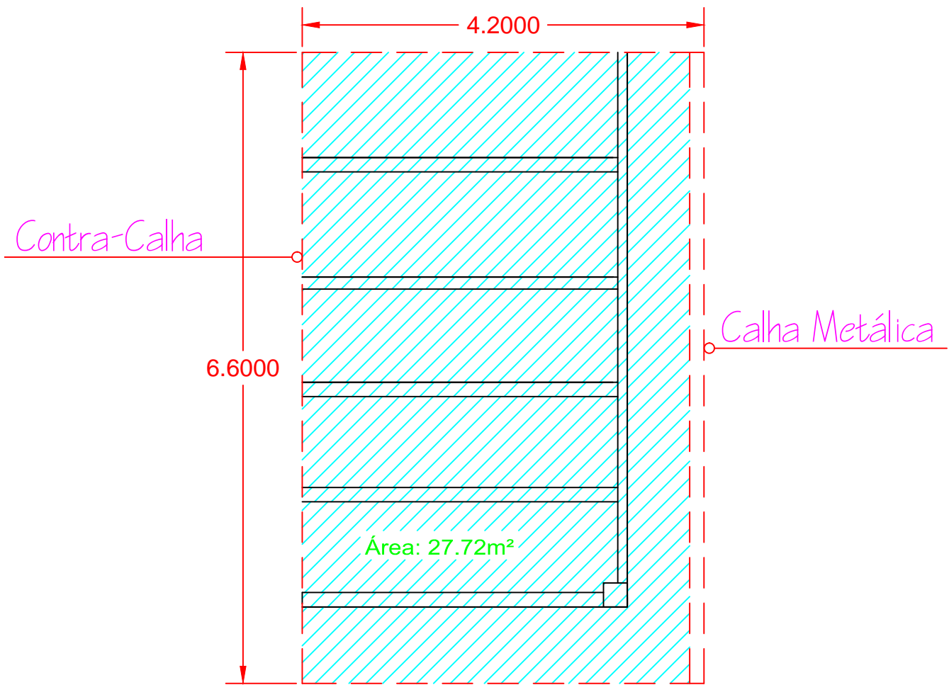
Planta Baixa Cobertura - Solarium 01 e 02
