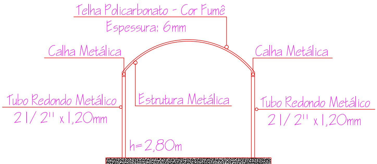
Vista Frontal - Rampa de Entrada
