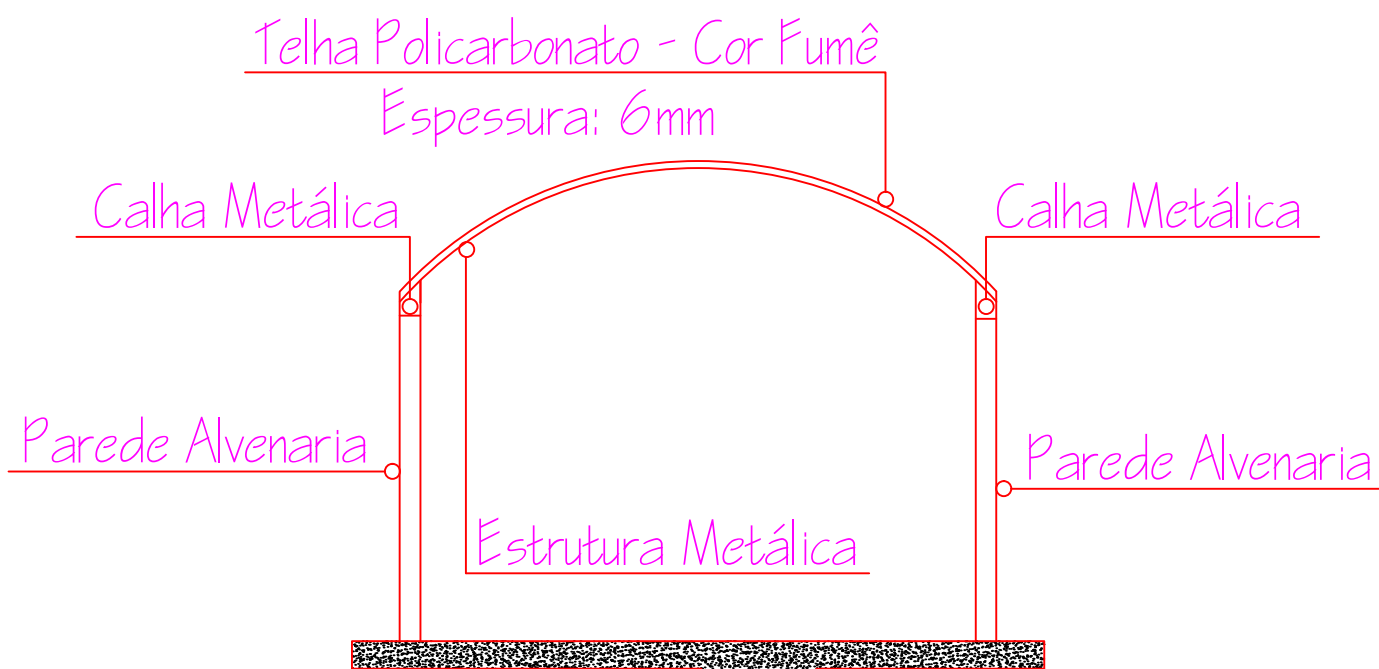
Vista Frontal - Entrada Pergolado
