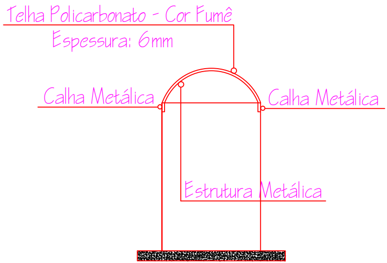
Vista Frontal - Toldo em "L" entre Prédios
