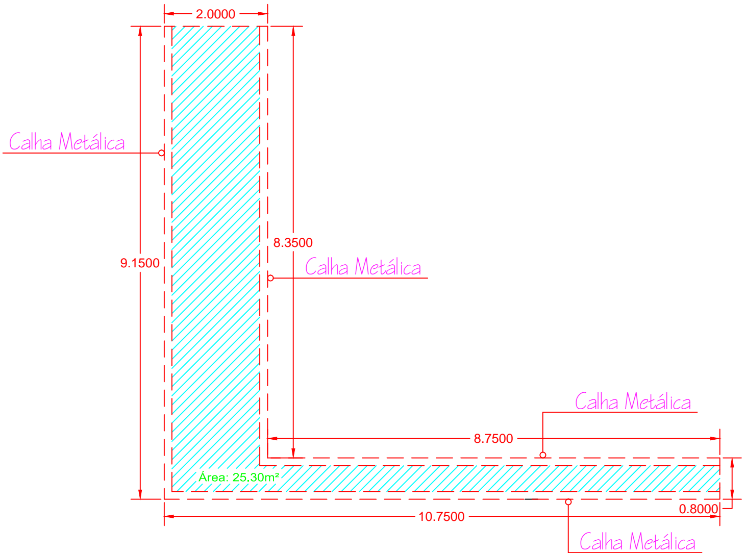
Planta de Cobertura - Toldo em "L" entre Prédios
