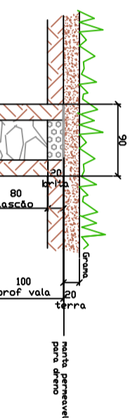
DETALHE VALA PERIFERICA SEM ESCALA
