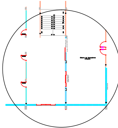
PORTA EXISTENTE DA CAMARA DE VEREADORES ( 2,30 M X 2,10 PORTA) E ( 2,30 X 0,90 CM DE VIDRO FIXO)
